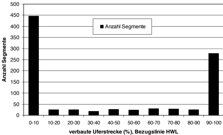
Abbildung 12: Häufigkeitsverteilung der 100 m-Segmente über dem klassierten Verbaungsgrad. Dargestellt ist die Zahl der Ufersegmente, die mit 0–10% usw. bis 90–100% ihrer Bezugslänge (HWL) verbaut sind.
