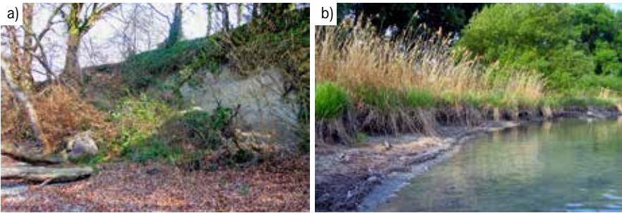
Abbildung 3: Unbefestigte Uferstrecken mit natürlicher Morphodynamik: (a) Geschiebekliff mit Hangrutschungen und Sturzbäumen (Mammern, Foto: 25.03.2011); (b) Seekreidekliff mit Röhrichtbestand am Seerhein-Ufer (Tägerwilen, Foto: 11.05.2011).
