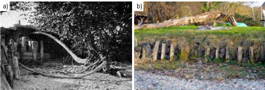
Abbildung 4: Mit einfachen Mitteln befestigte Uferabschnitte: (a) Stabilisierung eines Seekreidekliffs vor Streuwiesen bei Ermatingen im «Böschen» um 1907 ± 2 Jahre (aus Baumann 1911, Taf. I b); (b) mit Pfählen gesicherte Steinsetzung vor einer ehemaligen Streuobstwiese (aktuell extensiv genutzte Freizeit-Parzelle) bei Mammern (Foto: 25.03.2011).
