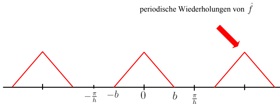
Figure 1: Der Shannonsche Abtastatz
