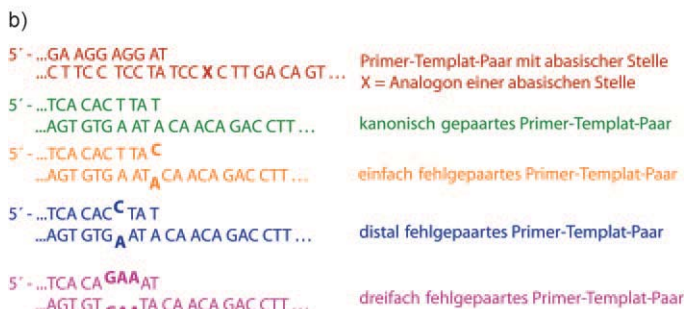
Abbildung 1. OAEA Prinzip. a) Kurze farbige Balken repräsentieren im immobilisierte Primer Stränge; lange farbige Balken repräsentieren Template, die selektiv durch die Hybridisierung mit den komplementären Primer Strängen adressiert werden. Grüne Sterne repräsentieren Streptavidin Alexa Fluor546 Konjugate, die an die eingebauten Biotine der verlängerten Primer Stränge binden. b) In dieser Studie verwendete Teilssequenzen.
