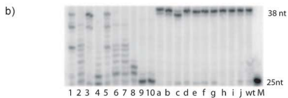
Abbildung 1. OAEA Prinzip. a) Kurze farbige Balken repräsentieren im immobilisierte Primer Stränge; lange farbige Balken repräsentieren Template, die selektiv durch die Hybridisierung mit den komplementären Primer Strängen adressiert werden. Grüne Sterne repräsentieren Streptavidin Alexa Fluor546 Konjugate, die an die eingebauten Biotine der verlängerten Primer Stränge binden. b) In dieser Studie verwendete Teilssequenzen.
