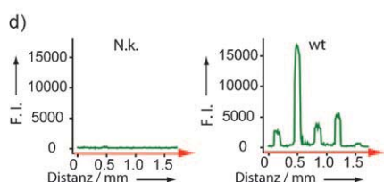
Abbildung 2. OAEA Evaluierung. a) Zehn zufällig ausgesuchte nichtaktive Mutanten (1-10) und zehn zufällig ausgesuchte aktive Mutanten (a-j). Eine genauere Betrachtung der Daten findet sich in den Hintergrundinformationen. b) Denaturierende Polyacrylamid Gelelektrophorese von in Lösung durchgeführten Primer Verlängerungsreaktionen durch die ausgesuchten Mutanten aus (a). M: Marker, Reaktion ohne Zellysate. c,d) OAEA Ergebnisse mit KlenTaq Wildtyp (wt) exprimierendem Zellysate und einer Negativkontrolle (N.k.) von Zellysaten mit einem Plasmid ohne das KlenTaq Gen. d) Fluoreszenz Intensitäts Profile (F.I.) entlang des roten Pfeils, wie in (c) angedeutet. Weitere experimentelle Details finden sich in den Hintergrundinformationen.
