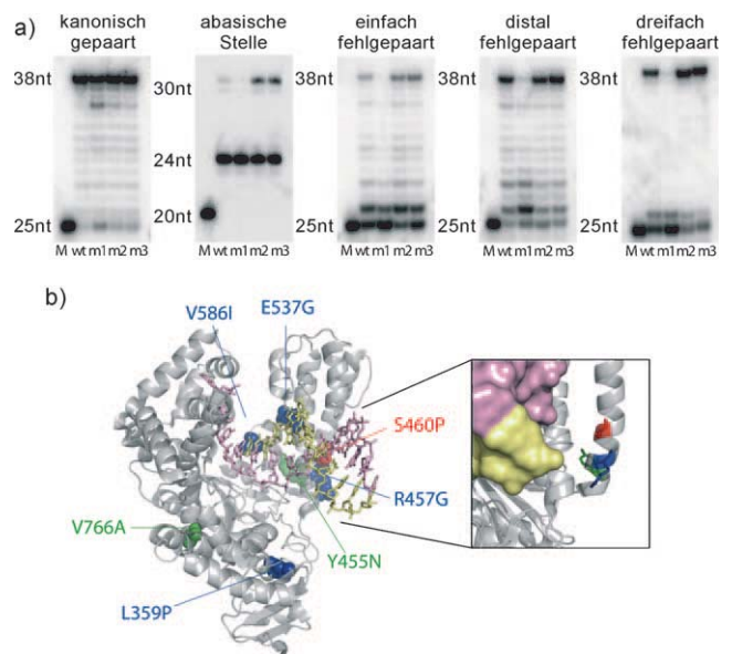
Abbildung 3. Evaluierung der veränderten Eigenschaften der durch OAEA identifizierten Mutanten. a) Prozessierung verschiedener DNA-Substrate in Lösung durch die evolvierten KlenTaq Mutanten (m1–m3) im Vergleich mit dem Wildtypenzym. Alle Reaktionen wurden mit den identischen Reaktionspuffer und dNTP-Konzentrationen durchgeführt (je 100 \mu M). Enzymkonzentrationen und Inkubationszeiten: kanonisch gepaart, einfach und distal fehlgepaart: 1 nM, 15 min; dreifach fehlgepaart und abasisch: 50 nM, 60 min. In den letzten beiden Fällen waren eine höhere Enzymkonzentration und eine verlängerte Inkubationszeit notwendig, um die Verlängerung der stärker gestörten DNA-Komplexe zu erzielen. Genauere experimentelle Details finden sich in den Hintergrundinformationen. M: Marker, Reaktion ohne Enzym. b) Die Mutationsstellen in den evolvierten KlenTaq DNA-Polymerasen m1 (rot), m2 (grün) und m3 (blau) sind in Form eines Bändermodells der KlenTaq (PDB-Code: 1QSS) [16] dargestellt. Die Vergrößerung zeigt die gefundenen Mutationsstellen von m1–m3 in der H-Helix.
