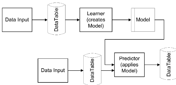
Abb. 2.: Skizze für einen Daten- und Modellfluss in KNIME.
