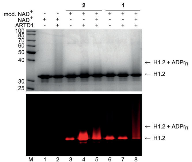
Abbildung 2. Vergleich der NAD + Analoga 1 und 2 mittels SDS PAGE Analyse der PARylierung von Histon H1.2. Oben: Coomassie Blue Färbung, Unten: TMR Fluoreszenz; Die NAD + Konzentration betrug 1 mM. Kontrollreaktionen wurden mit natürlichem Substrat (Bahn 1 und 2) sowie ohne Zugabe von Enzym (Bahn 3 und 6) durchgeführt. Jedes Analogon wurde auch in einem 1:1 Gemisch mit natürlichem NAD + untersucht (Bahn 5 und 8).
