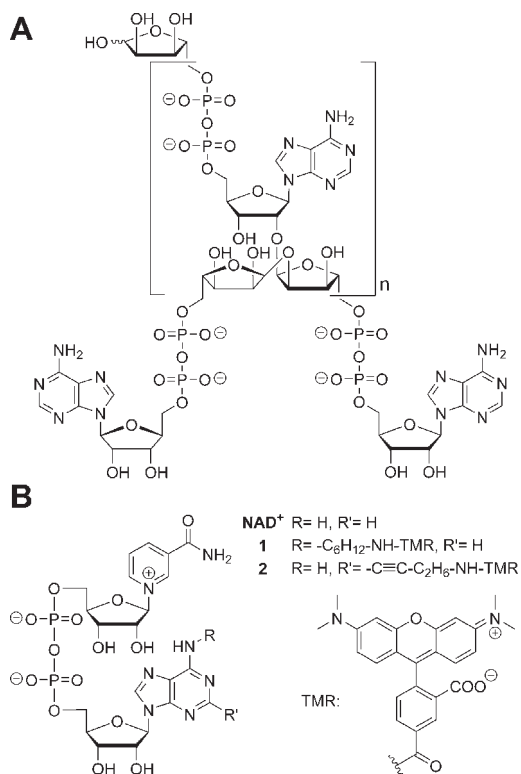
Abbildung 1. Struktur von A) Poly(ADP ribose) und B) NAD + und NAD + Analoga 1 und 2 , die in dieser Studie verwendet wurden.
