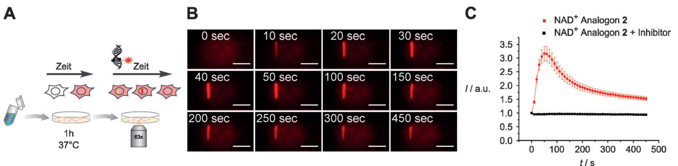
Abbildung 4. Beobachtung von PARylierung nach DNA Schädigung in lebenden Zellen mithilfe des NAD + Analogons 2 . A) Experimenteller Aufbau. HeLa Zellen werden mit 2 beladen und zur DNA Schädigung mikrobestrahlt. B) Exemplarische Sequenz der konfokalen Mikroskopiebilder. Maßstab: 7 μm. C) Quantitative Analyse der relativen Fluoreszenzverstärkung am Ort des DNA Schadens im Vergleich zur Umgebung ( n = 32 Zellen). Kontrollexperimente wurden mit 10 μM ARTD Inhibitor ABT888 ( n = 28 Zellen) durchgeführt. Drei unabhängige Experimente wurden durchgeführt. Fehlerbalken entsprechen dem Standardfehler (SEM).
