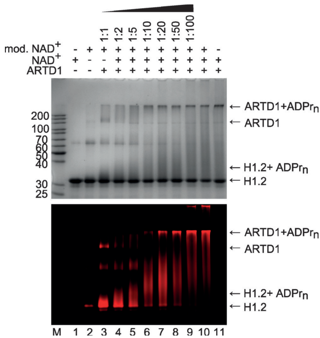
Abbildung 3. SDS PAGE Analyse der PARylierung von Histon H1.2 mit NAD + Analogon 2 und natürlichem NAD + . Oben: Coomassie Blue Färbung; unten: TMR Fluoreszenz. Die NAD + Konzentration betrug 1 mM mit angegebenen Verhältnissen von modifizierten zu unmodifizierten NAD + . Kontrollreaktionen wurden mit natürlichem Substrat (Bahn 1 und 11) sowie ohne Zugabe von Enzym (Bahn 1 und 2) durchgeführt.
