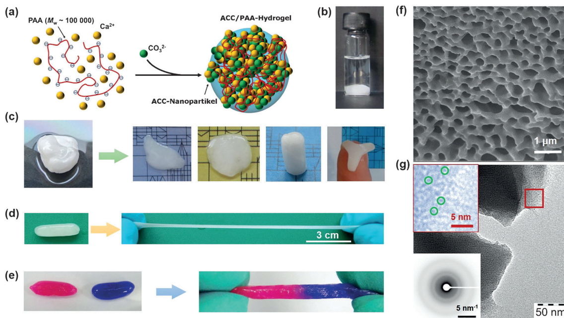
Abbildung 1. (a) Schema der Synthese des supramolekularen ACC/PAA Hydrogels. (b) Das ACC/PAA Hydrogel ist in Wasser stabil. (c) Das Hydrogel ist plastisch und kann in verschiedene Formen gebracht werden. (d) Es ist außerdem dehnbar. (e) Selbstheilendes Verhalten des ACC/PAA Hydrogels. Zur Verdeutlichung wurden die Hydrogele mit Farbstoffen (Rhodamin B und Methylblau) eingefärbt. (f) SEM Aufnahme des gefriergetrockneten Hydrogels. (g) TEM Aufnahme des getrockneten Gels. Eingefügt sind ein Elektronenbeugungsdiffraktogramm sowie eine vergrößerte Ansicht des rot umrandeten Bereichs, die die Anwesenheit kleiner ACC Partikel zeigt (grün umrandet).
