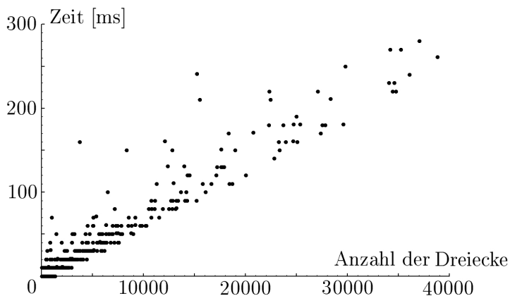
Abb. 11: Scatter Plot für die Zeitkomplexität der Berechnung der Parameter der modifizierten Karhunen-Loeve Transformation zur Berechnung der kanonischen Lage und Orientierung
