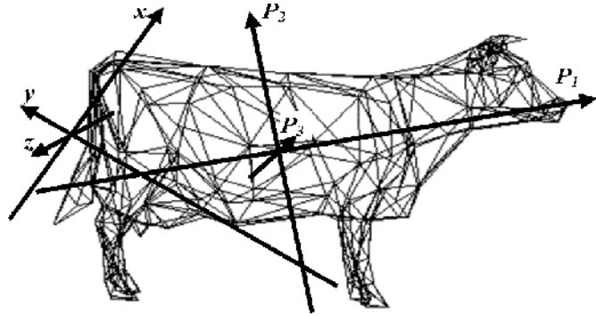
Abb. 4: Die modifizierte Karhunen-Loeve-Transformation angewendet für ein Modell
