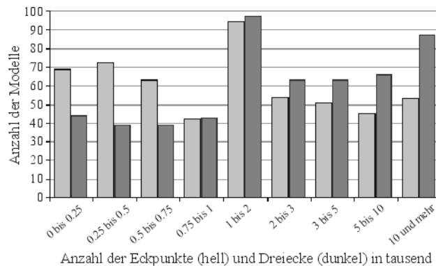
Abb. 10: Histogramm für die Modellkomplexität
