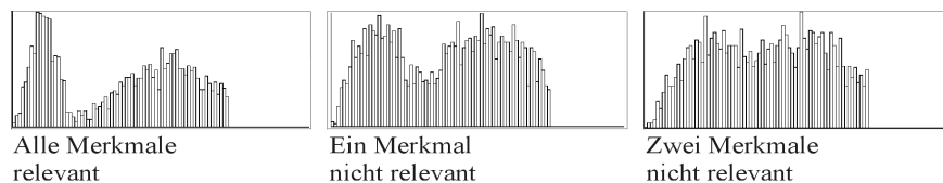
Abb. 2: Die Distanz-Verteilung bei unterschiedlicher Anzahl relevanter Merkmale
