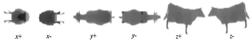
Abb. 8: Sechs Tiefenpuffer
