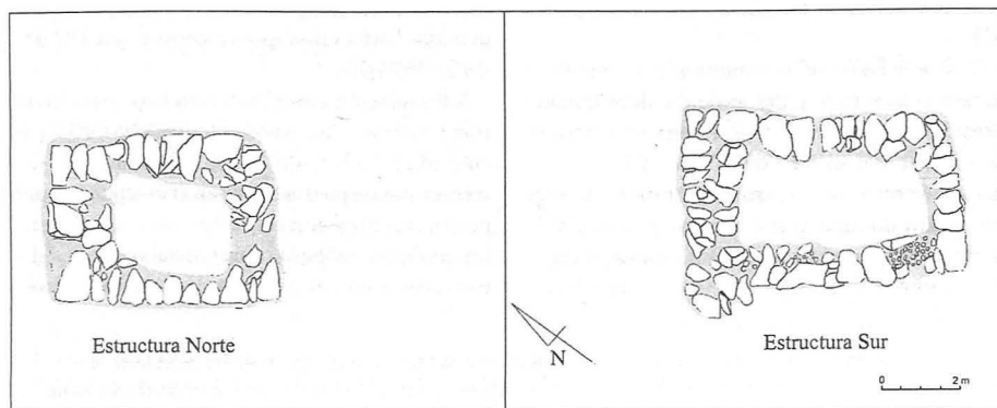
Figura 9. Dibujo de planta de las estructuras excavadas en el sitio PV67A-80.
