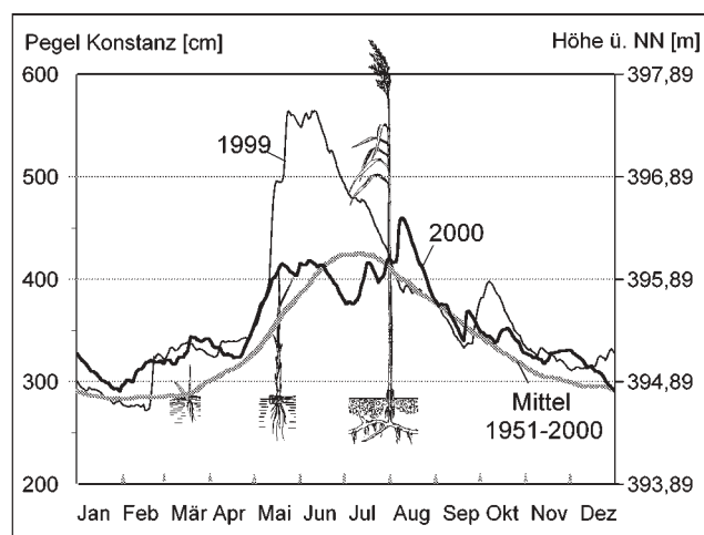
Abb. 2. Mittlere Wasserstandsganglinie 1951–2000 und Wasserstandsganglinien für die Jahre 1999 und 2000 am Pegel Konstanz (Bodensee-Obersee). Die drei Schilfpflanzen sind in Größe und Höhenlage maßstabsgerecht eingezeichnet.
