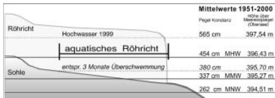
Abb. 3. Schema eines Schilfröhrichts am Bodensee-Obersee mit den Hauptzahlen des Konstanzer Pegels für den Zeitraum 1951 bis 2000. Für den Untersee muss bei den Höhenwerten über Normalnull 0,19 m abgezogen werden.
