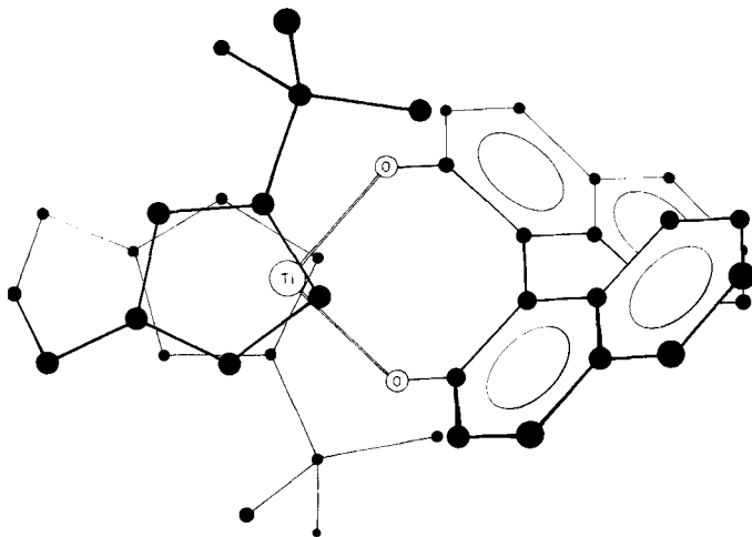
Abb. 1. Molekülmodell von 1 S ,1' S -Trimethylen-bis(3- tert -butylcyclopentadienyl)titan(IV)-(S)-1,1'-Bi-2-naphtholat (2) (Projektion auf \text{TiO}_2 -Ebene, Höhenlage der C-Atome durch Größe der dunklen Kreise angedeutet) [8].
